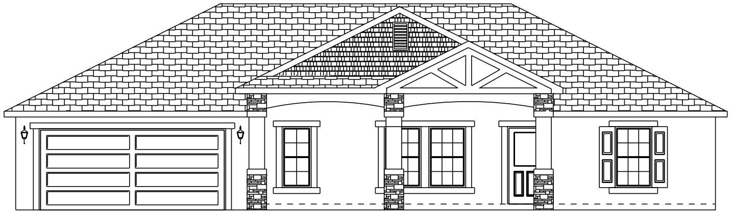
ELEVATION A
